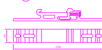
③ 딘레일 브라켓
