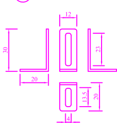
② ㄱ자 브라켓
